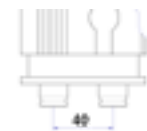
S-Line® GSP-System für Rundloch- Ankerschienen mit 40 mm Raster
